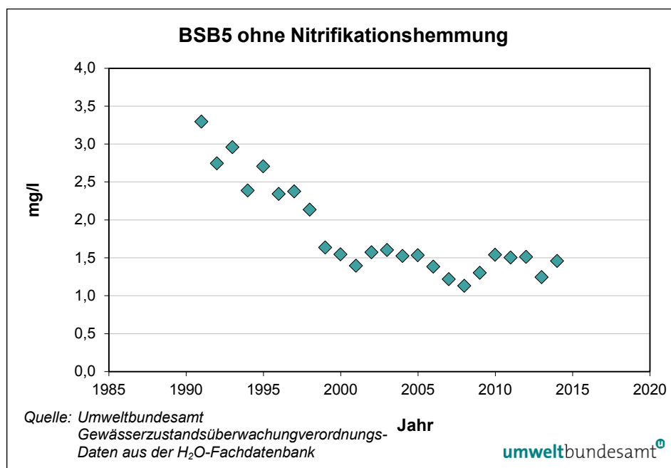
Abbildung 18: Trend des BSB5 ohne Nitrifikationshemmung. Dargestellt sind die gesamtösterreichischen Mittelwerte der 90 % Perzentilen für jene 36 Fließgewässer- Einzelstandorte mit durchgehenden Zeitreihen von 1992–2014.
